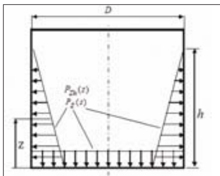
Рис. 3. Гидродинамическое давление на стенки и днище от вертикального сейсмического воздействия
