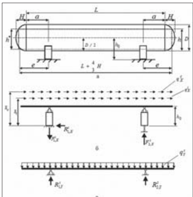
Рис. 4. Расчетная модель горизонтального сосуда
