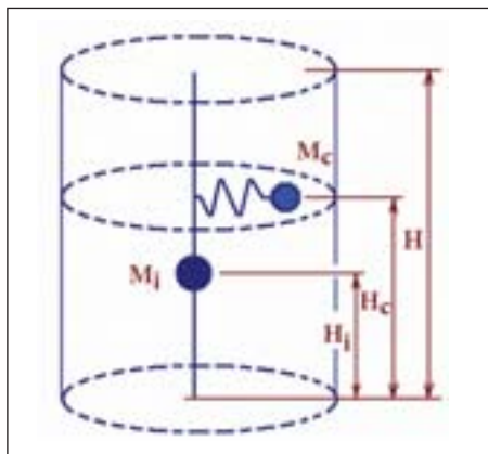
Рис. 1. Расчетная модель вертикального цилиндрического резервуара с жидкостью
