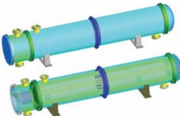
Рис. 5. Расчетная модель горизонтального сосуда
